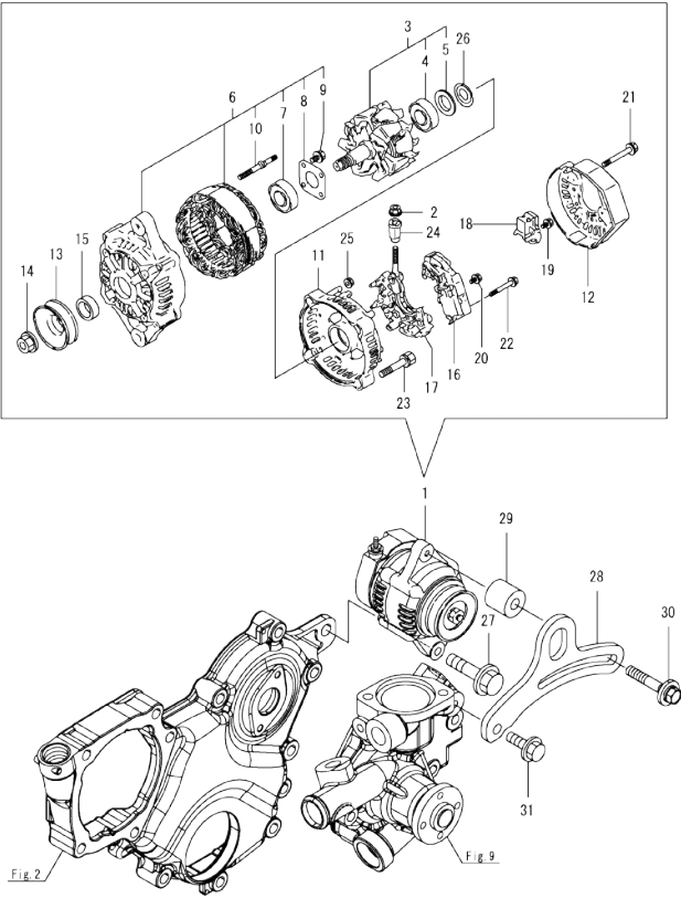
Fig.15. GENERATOR
